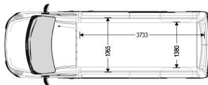
WYMIARY POWIERZCHNI ŁADUNKOWEJ
