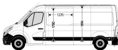
WYMIAR DRZWI BOCZNYCH PRZESUWANYCH / WYSOKOŚĆ PRZESTRZENI ŁADUNKOWEJ
